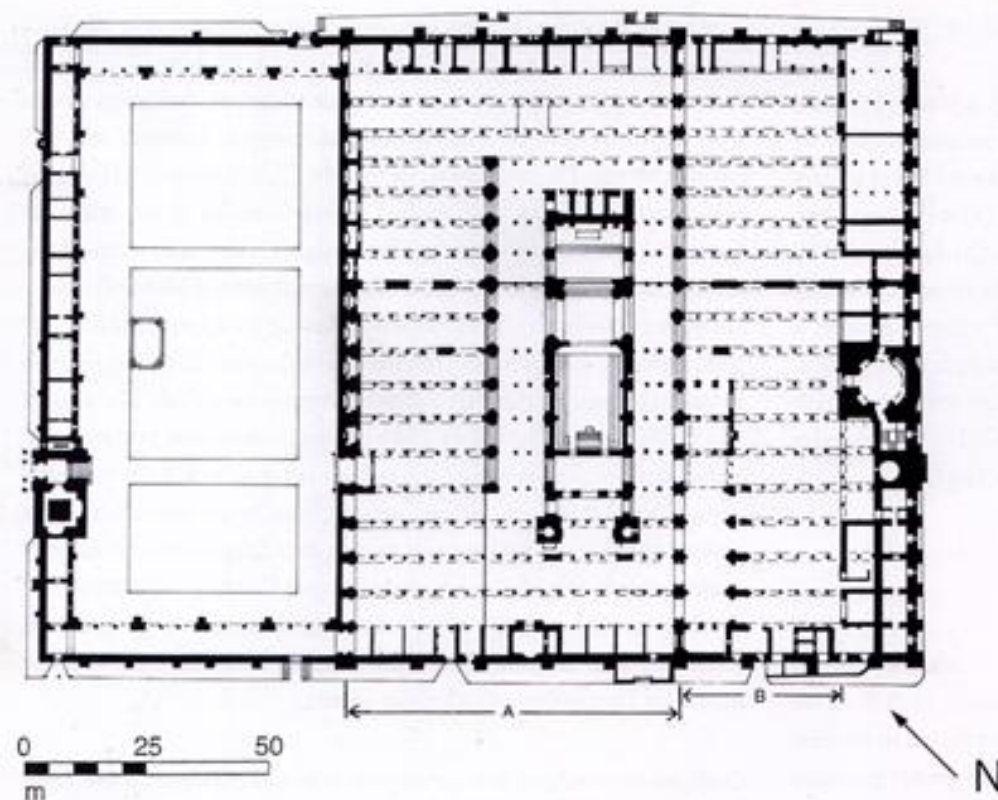
Planta da Grande Mesquita de Córdoba, em sua forma final. A dimensão da mesquita original (A). Diagrama (acima) que indica o método de cálculo utilizado no acréscimo realizado no século IX.
